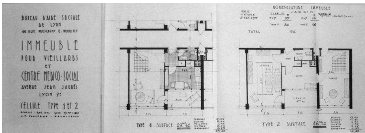
Plan des cellules types 1 et 2, immeuble pour vieillards et centre médico-social, 13 mai 1960 par J.P. Fonterme architecte, échelle 1/50. (Arch. mun. Lyon)
