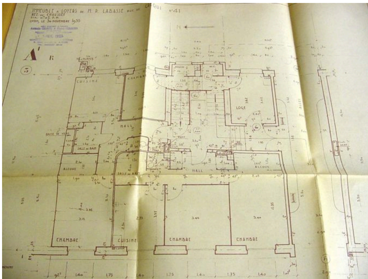
41 rue de Créqui. Plan du rez-de-chaussée / Verrier et Chomel, 1935
