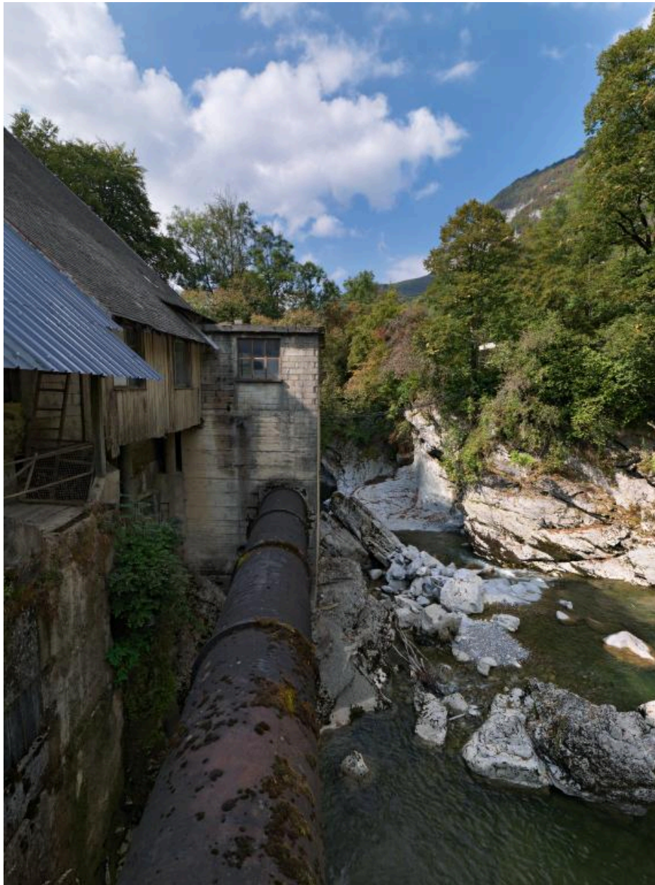
Conduite forcée de la micro-centrale électrique de la scierie Dagand.
