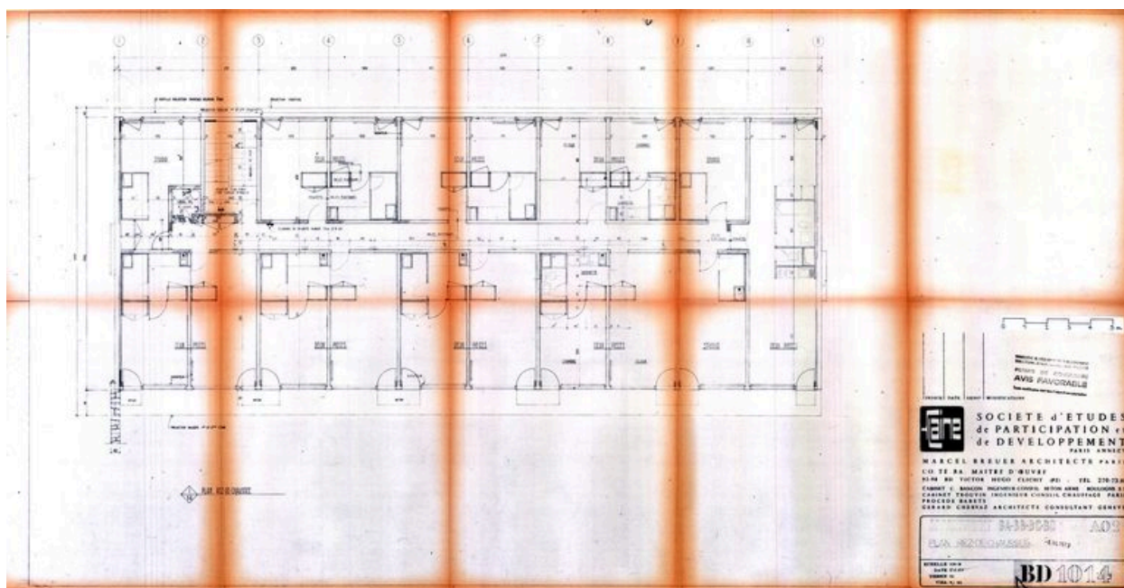
Plan du rez-de-chaussée. Marcel Breuer architecte, 27 février 1973 (AC Magland)
