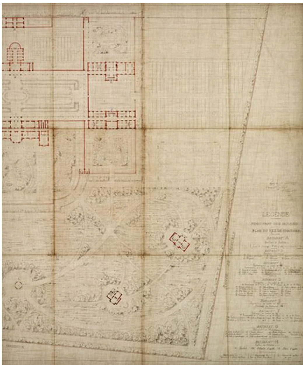
Antonin Louvier, pensionnat des hommes, plan du rez-de-chaussée, 10 novembre 1877 : détail de la partie droite, avec légende
