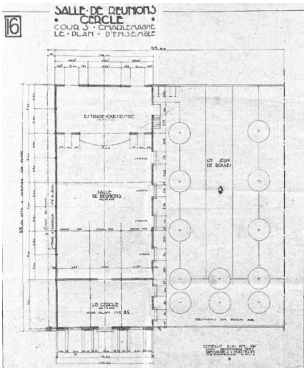
Plan d'ensemble, 1927
