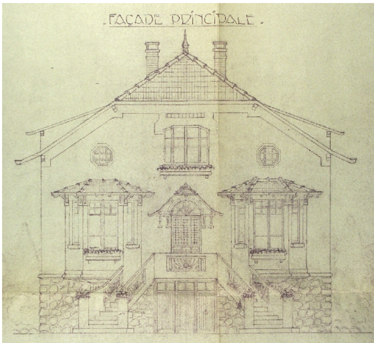
Elévation principale
