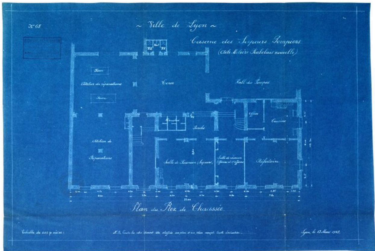
Plan du rez-de-chaussée, 13 mars 1923
