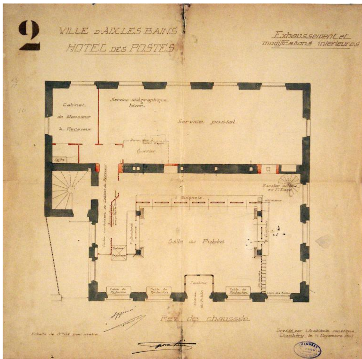
Exhaussement et modifications intérieures, 1907 : plan du rez-de-chaussée
