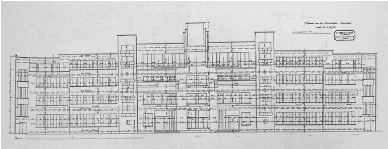
Façade sur l'avenue Jean-Jaurès, Réalisation Ecole primaire de Gerland, 2 aout 1932 par V.-A. Robert et A.-E. Chollat architectes, échelle 1/100. (AC Lyon)
