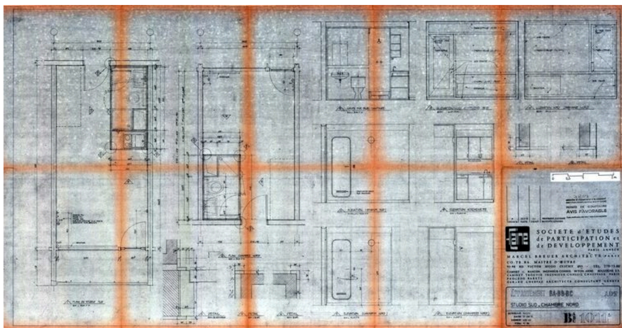
Studio sud, chambre nord. Plan, élévations, détails. Marcel Breuer architecte, 27 novembre 1972. Modifié le 27 février 1973 (AC Magland)
