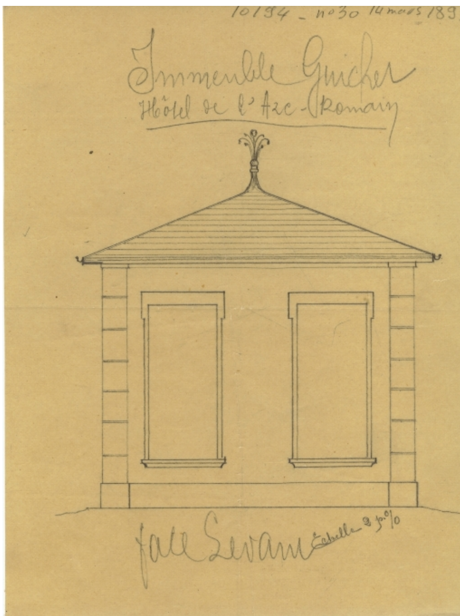
Elévation orientale de la salle à manger
