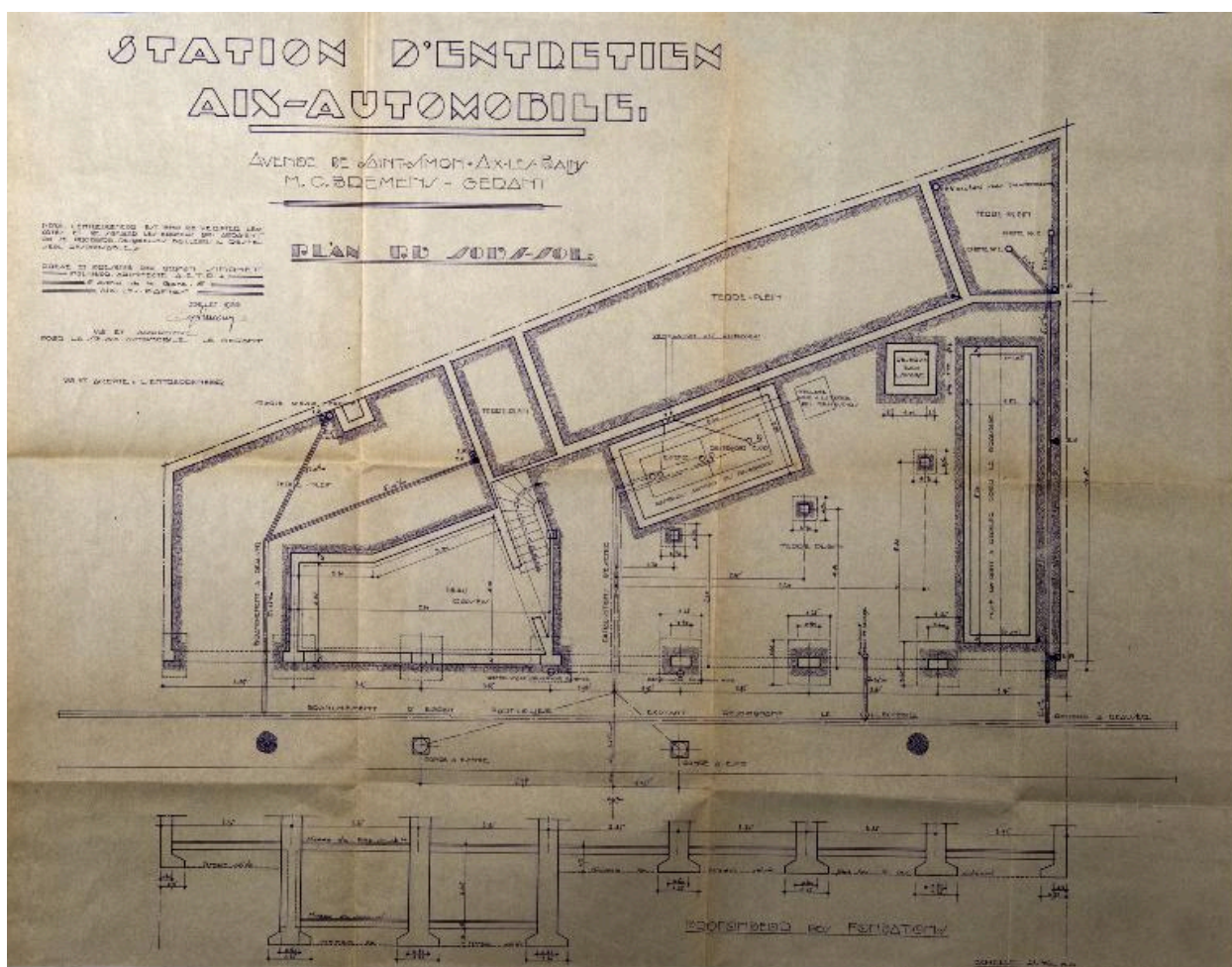
Plan du sous-sol, 1930
