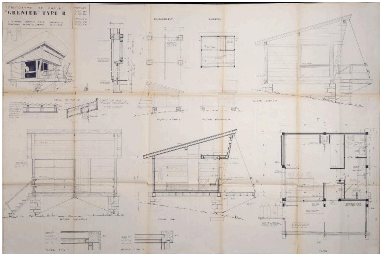
Chalet type B ou modèle Lilliput : plans, coupes et élévations, 1954
