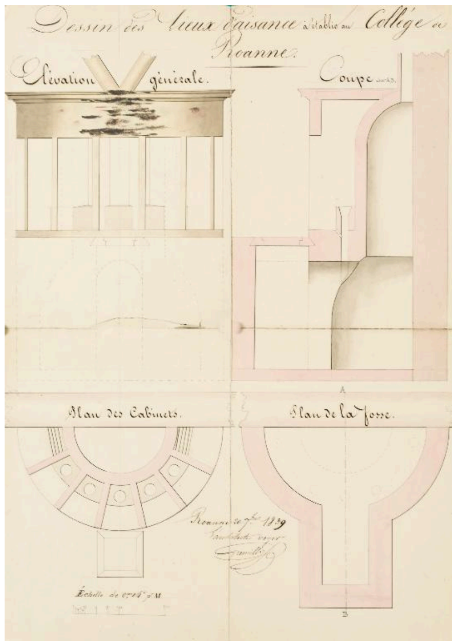
Plan : Dessin des lieux d'aisance à établir au collège de Roanne. (1839)
