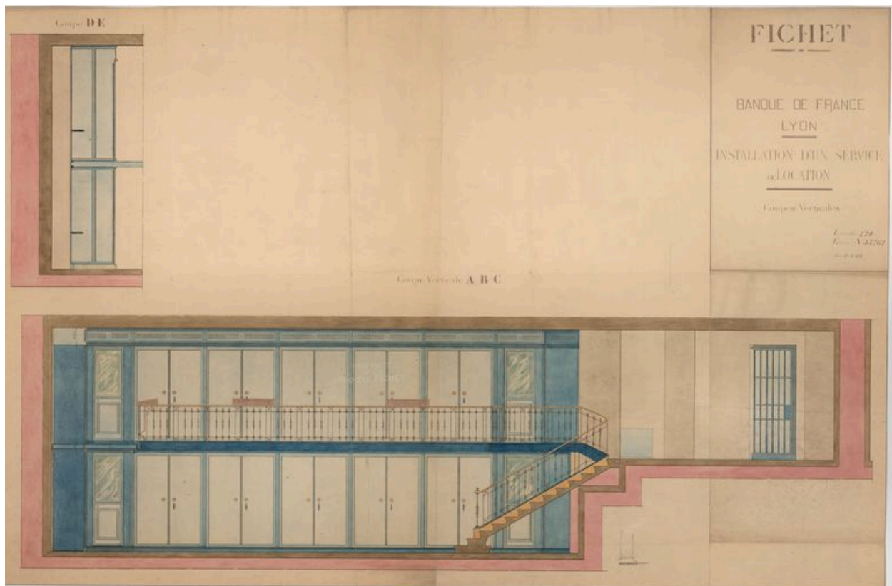
Coupe (aquarellée) sur la salle des coffres aménagée par Fichet (1922) (Banque de France, service du Patrimoine Historique et Artistique, non coté, dessin).
