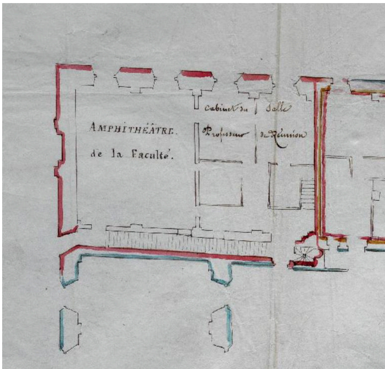
Plan de distribution, 1er étage, ca 1849 (détail)
