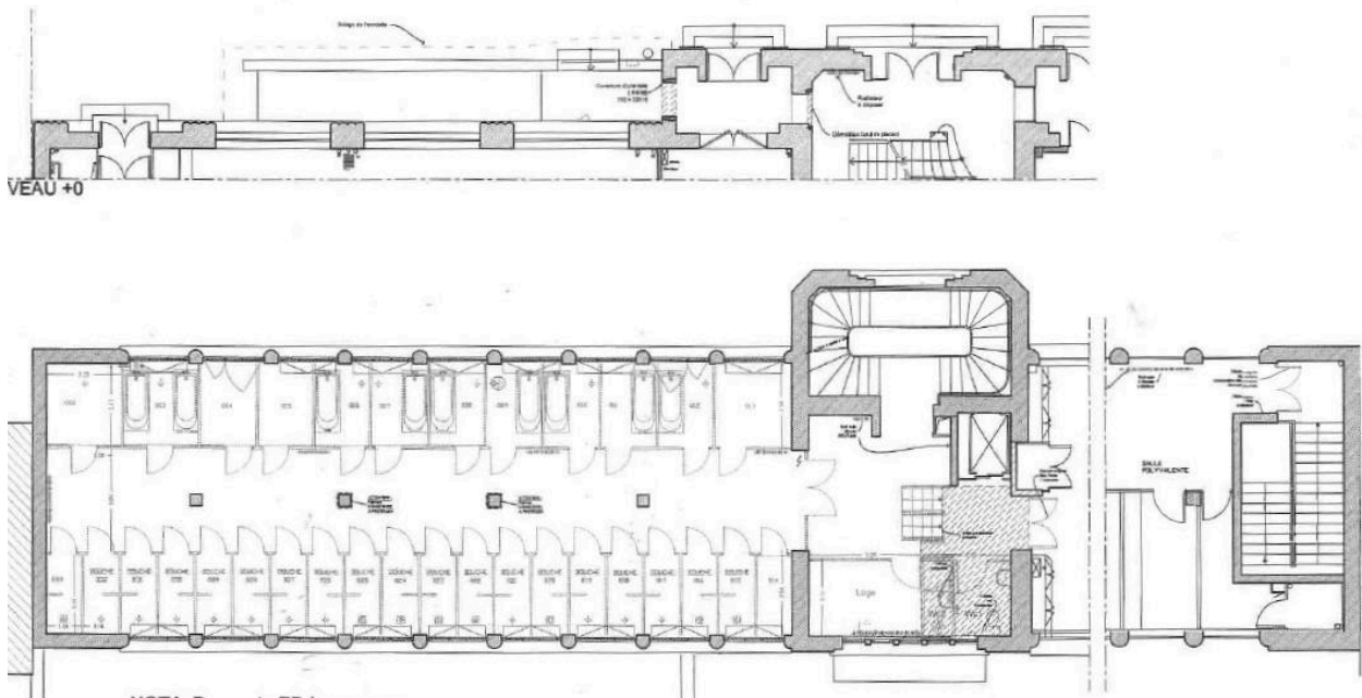
Plan des bains-douches niveau 1 (archives SAAL)
