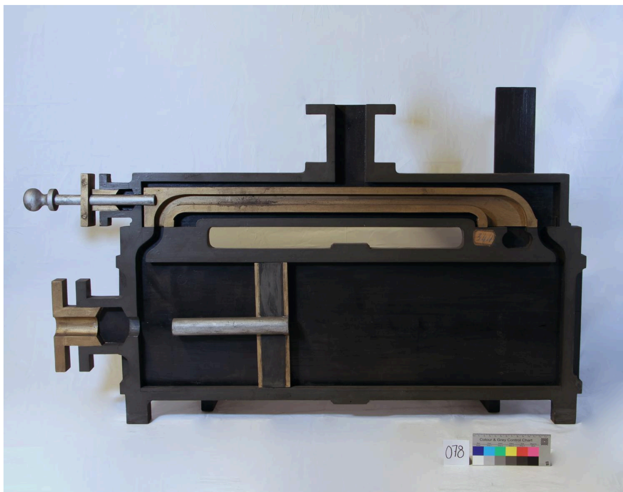
Modèle de piston, vue de face
