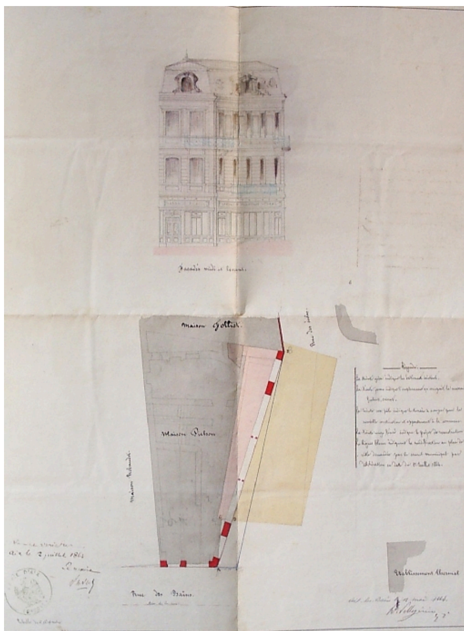
Plan d'alignement et élévation
