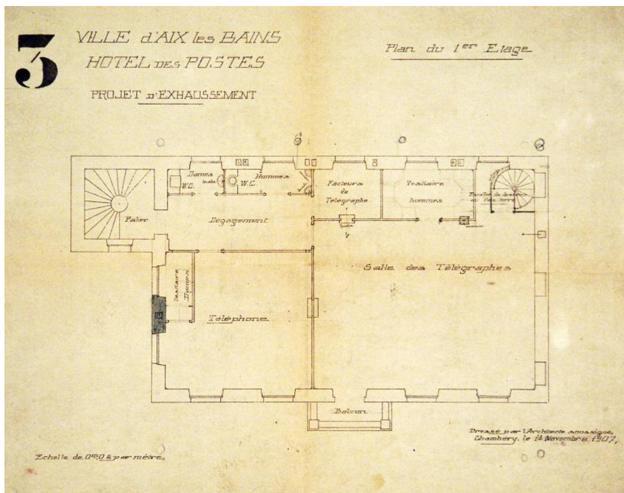
Exhaussement et modifications intérieures, 1907 : plan du 1er étage
