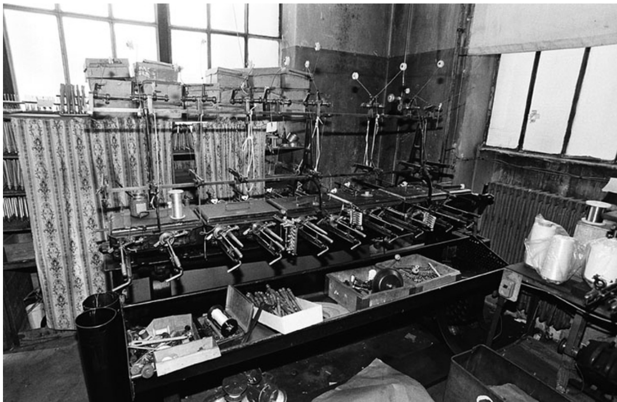
Cannetière à grande production modèle CK
