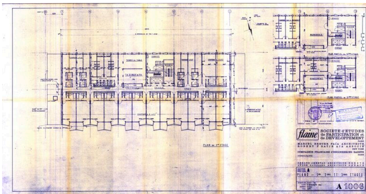
Hôtel A. Plan des 1er, 3e et 5e étages. Marcel Breuer architecte, Robert F. Gatje associé, 7 novembre 1961. Révision générale 12 décembre 1961 (AC Arâches-la-Frasse)
