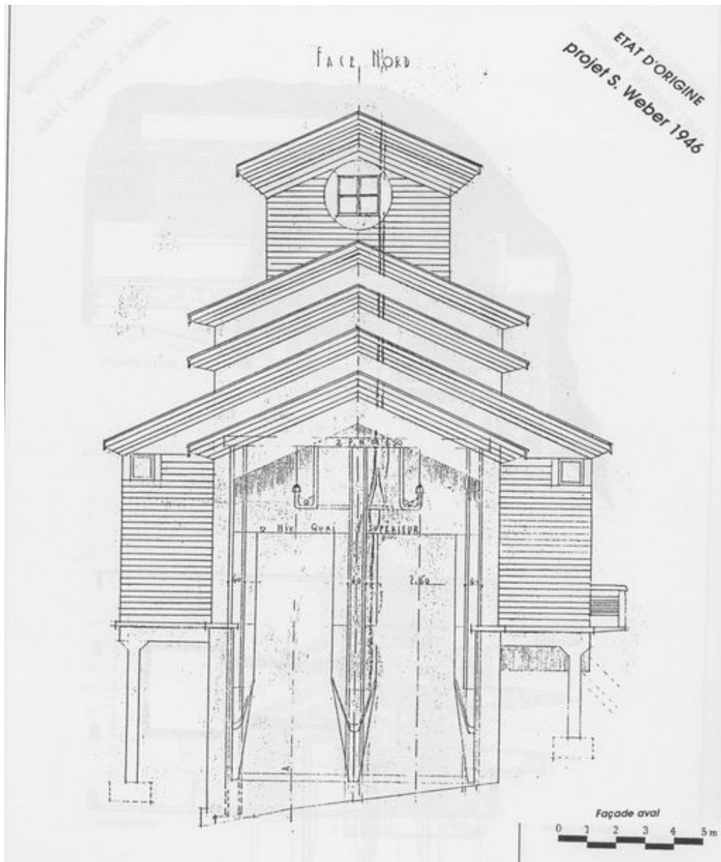
Gare supérieure. Elévation nord. Projet / Stéphane Weber, 1946
