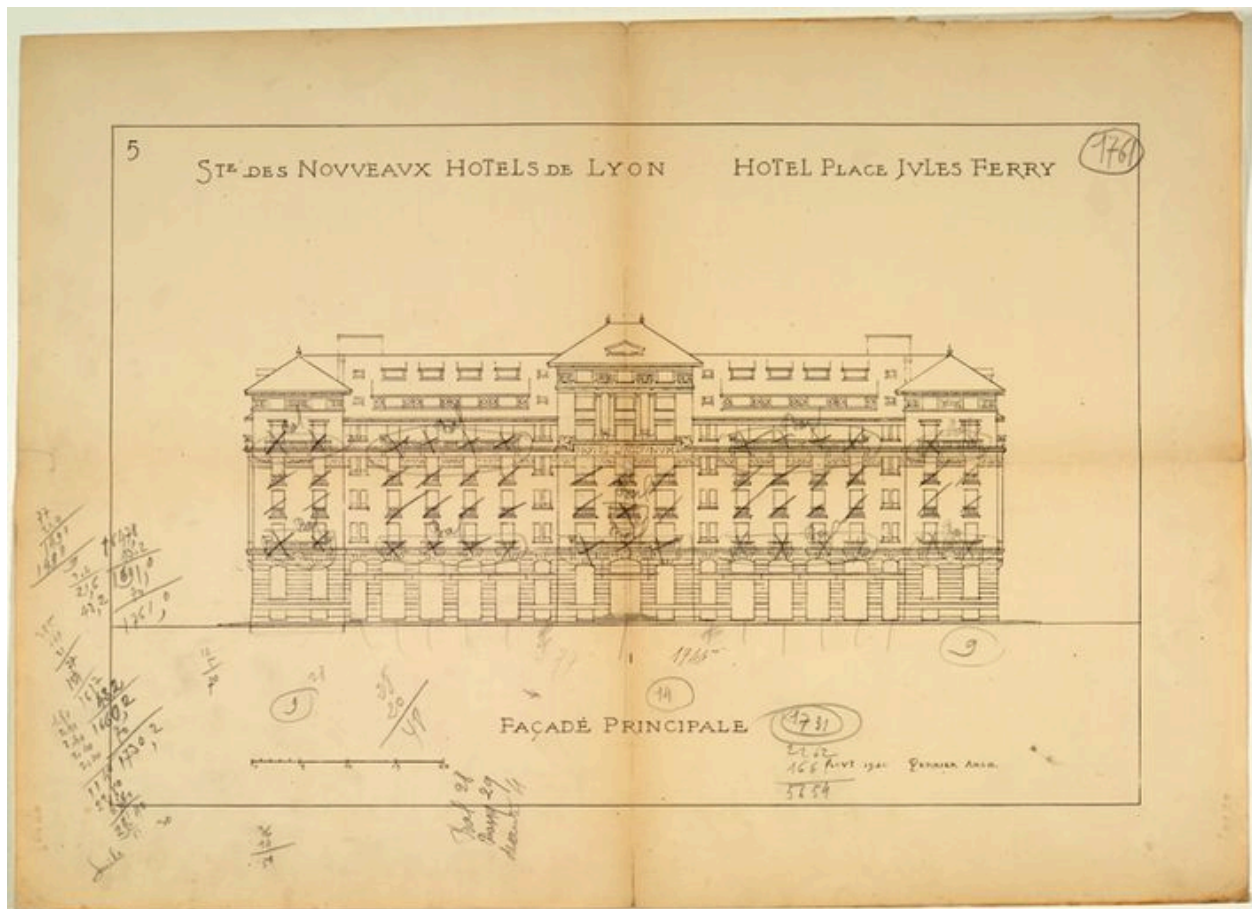
Élévation antérieure, Valère Perrier architecte, 1920
