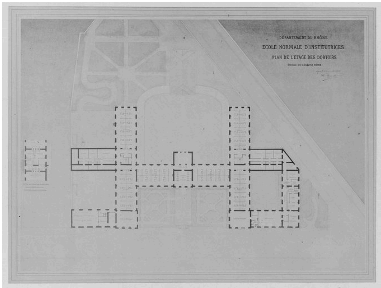
Plan du premier étage de l'école normale (étage dit des dortoirs, 1888) (Arch. dép. Rhône, 1 T 1267, photographie de Fernique).
