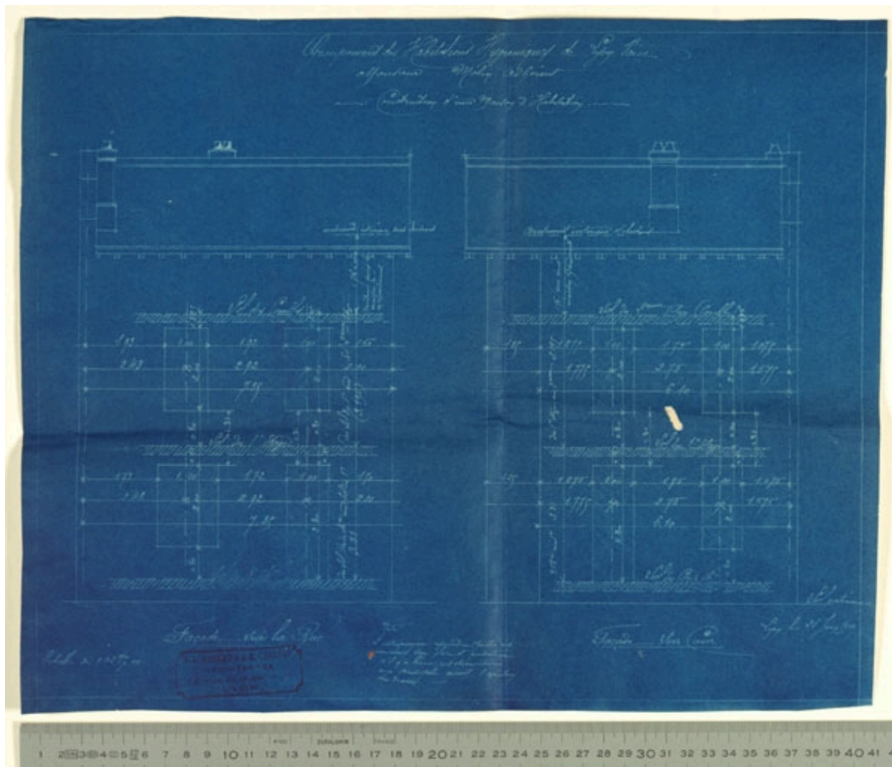
314 WP 1910 permis 487, façades d'une maison individuelle au 28 rue Littré
