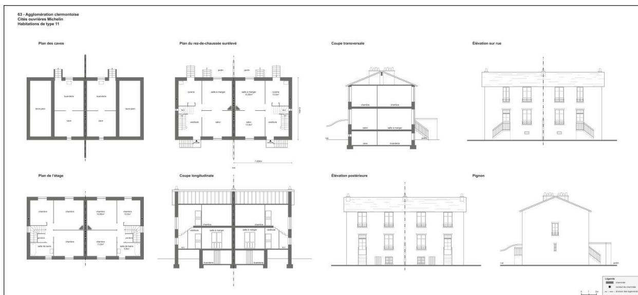
Plan des habitations d'employés de type 11.
