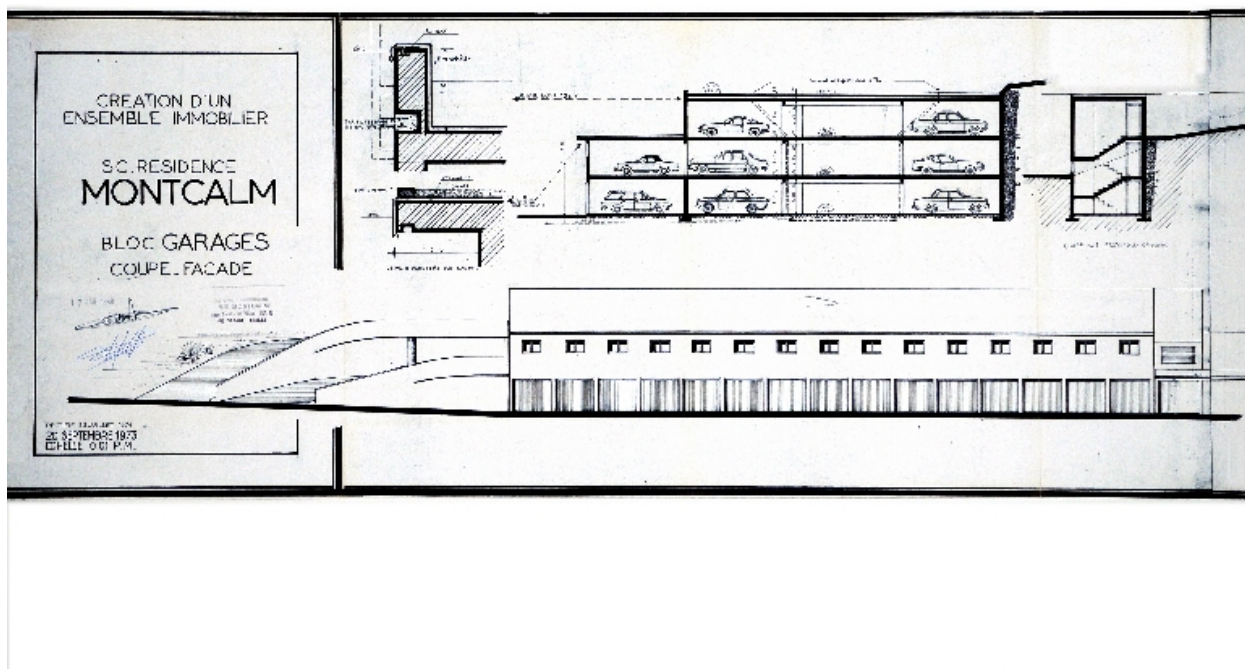
Coupe et élévation des garages
