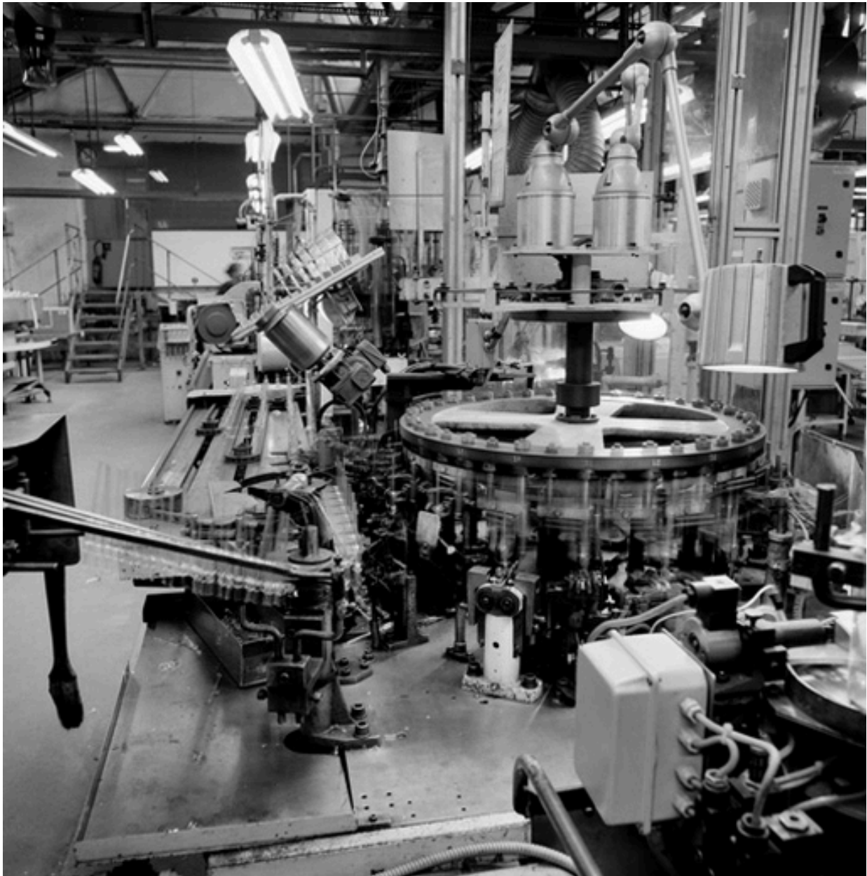
Vue d'ensemble de la ligne de montage
