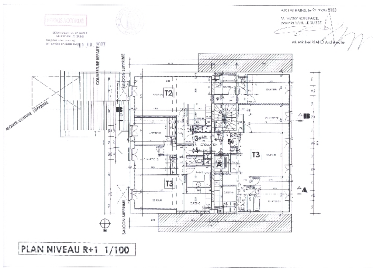
Plan du premier étage après transformation
