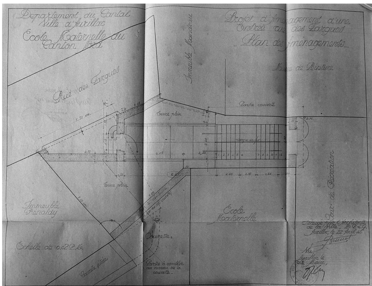
Projet d'aménagement de l'entrée rue des Fargues : plan des aménagements par J. Brunot, 1945 (AD Cantal, E DEP 1500/1506)
