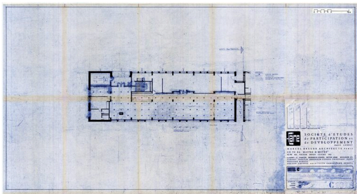
Hôtel C. Projection du plafond du rez-de-chaussée. Marcel Breuer architecte, 30 octobre 1967. Modification 7 février 1968 (AC Arâches-la-Frasse)
