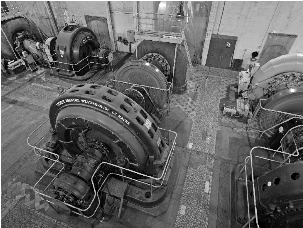
Vue d'un groupe de la centrale de Livet
