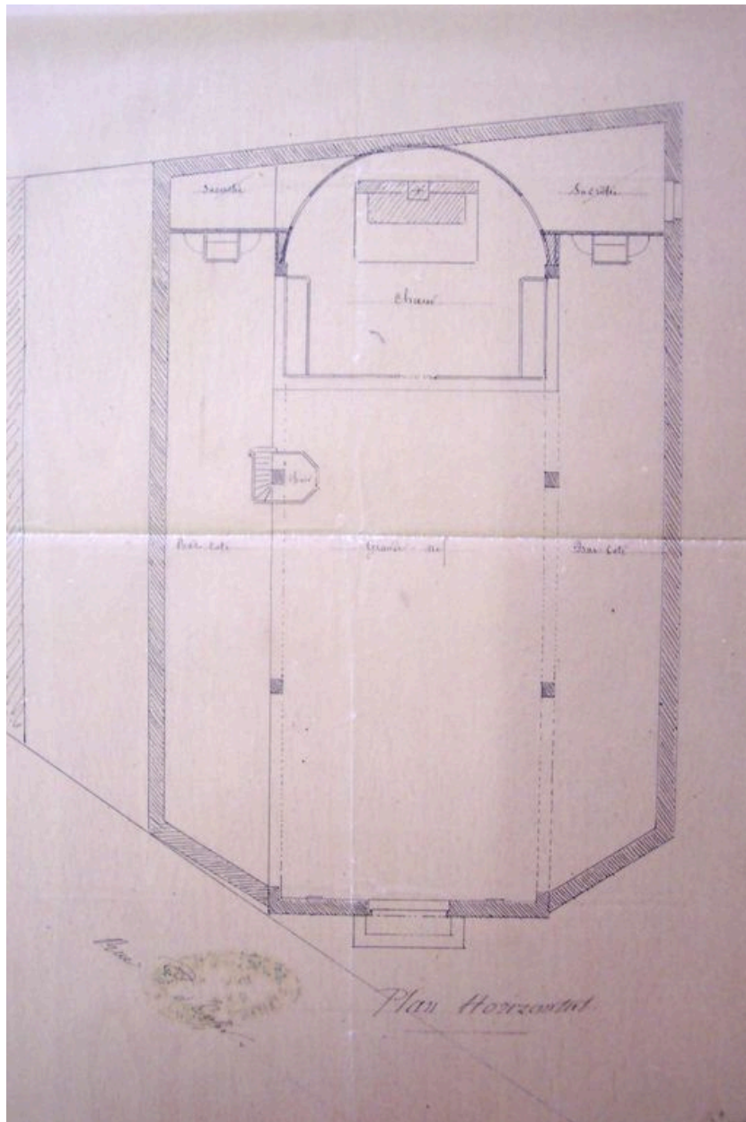
Plan général de l'église par l'architecte Bourdet
