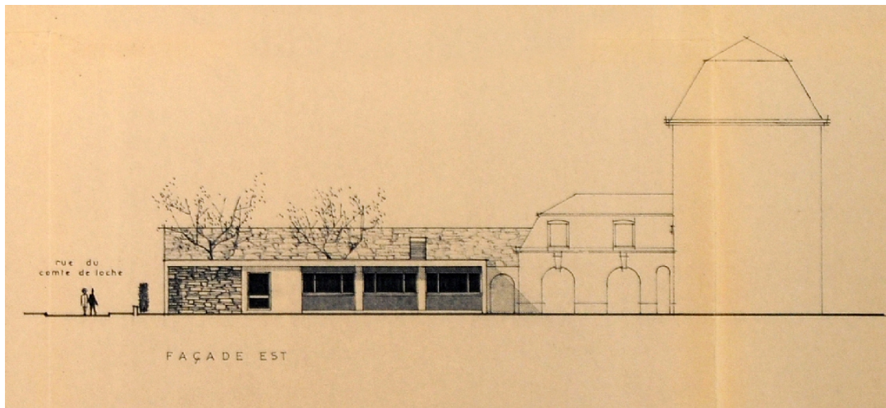
Façade est
