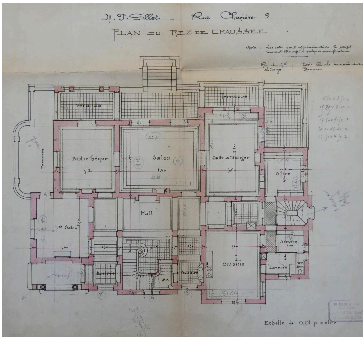
Plan du rez-de-chaussée 1911 (AC Lyon314W435-558)
