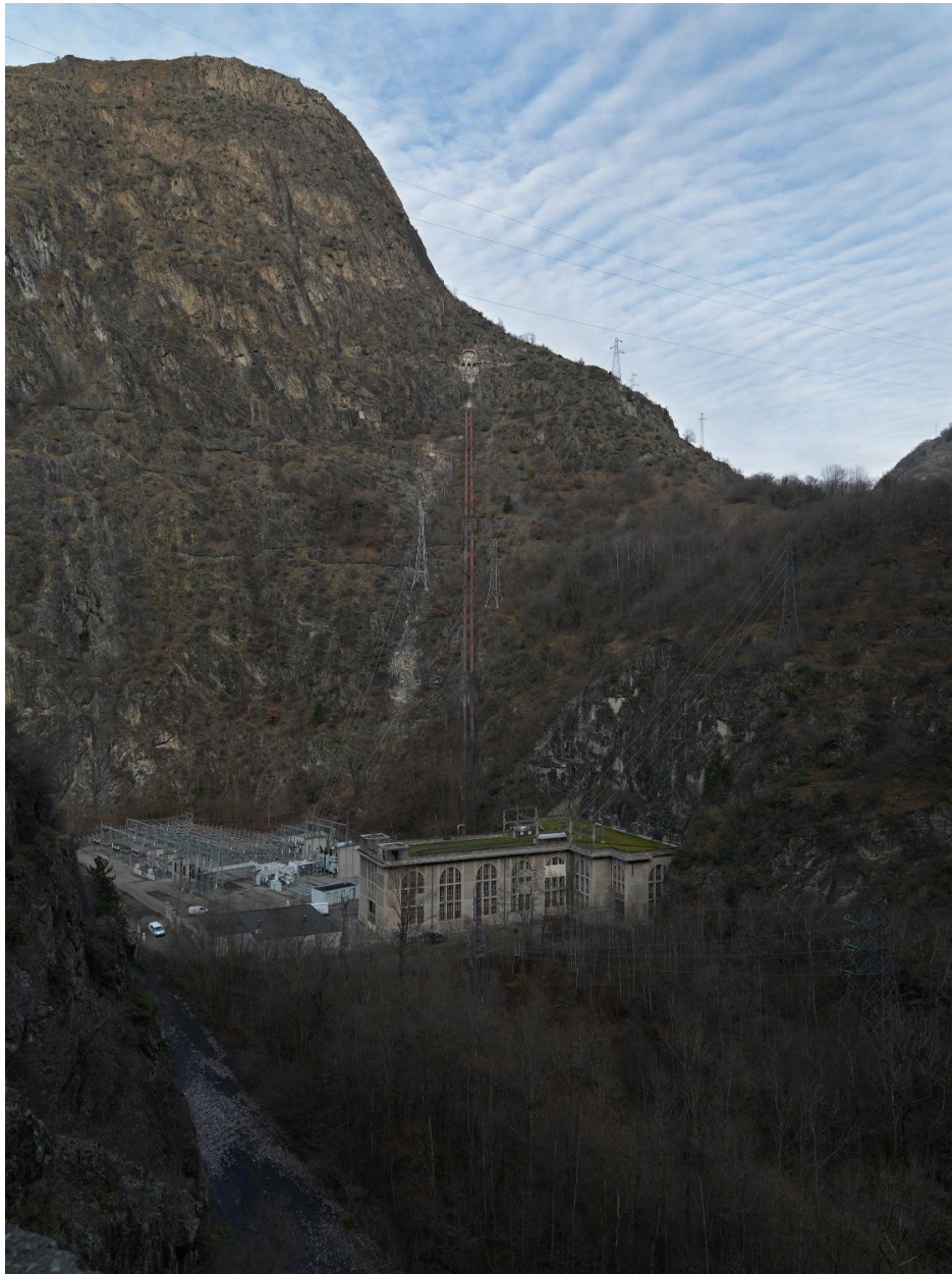
Vue d'ensemble de la centrale de Saint-Guillaume I avec conduites forcée et chambre de mise en charge.
