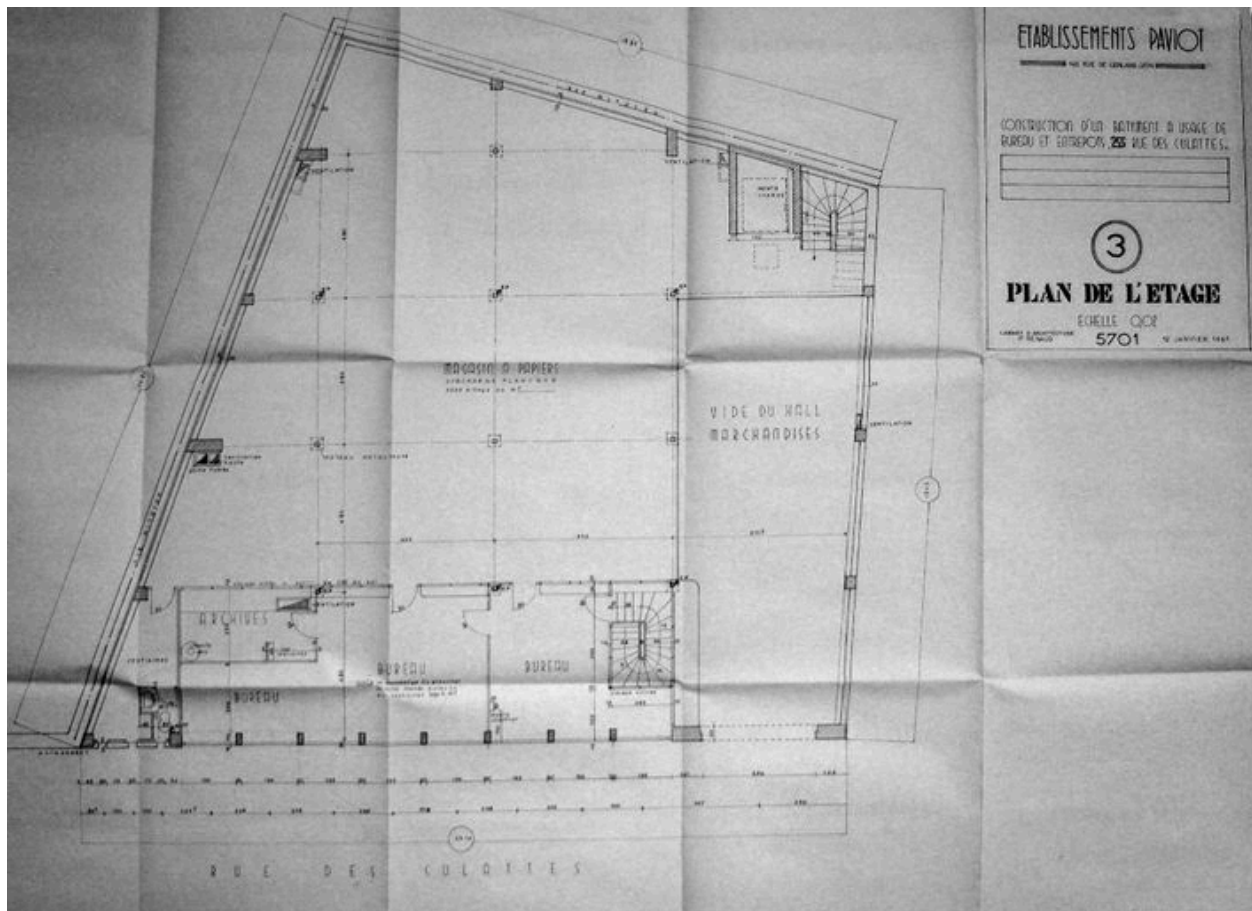
Plan de l'étage, 255 rue des Culattes, 20 janvier 1961 par Pierre Renaud architecte, échelle 1/50. (Arch. mun. Lyon)
