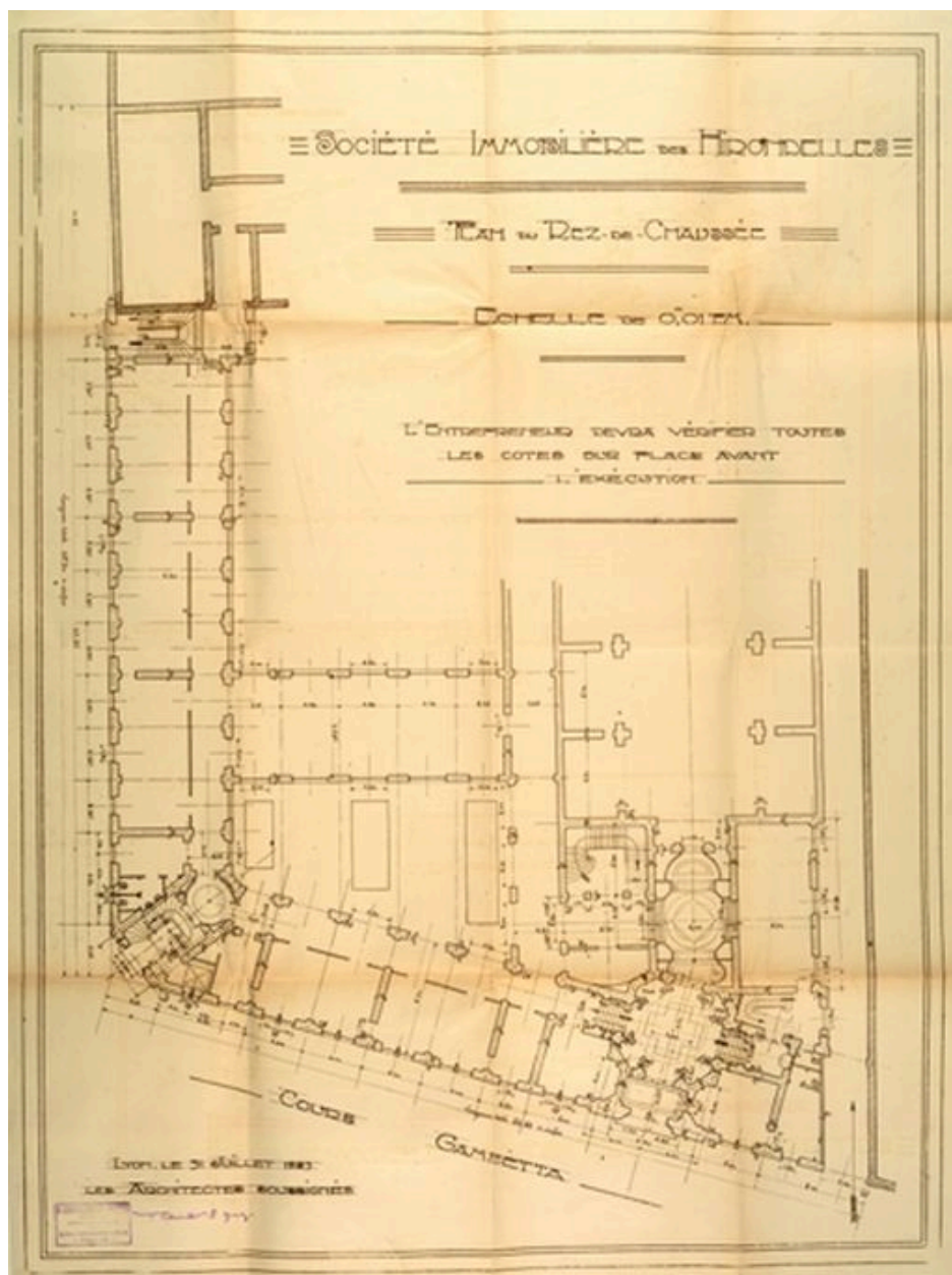
Plan du rez-de-chaussée / F. Chevallet et E. Martin, 1923 (AC Lyon. 344 WP 134)
