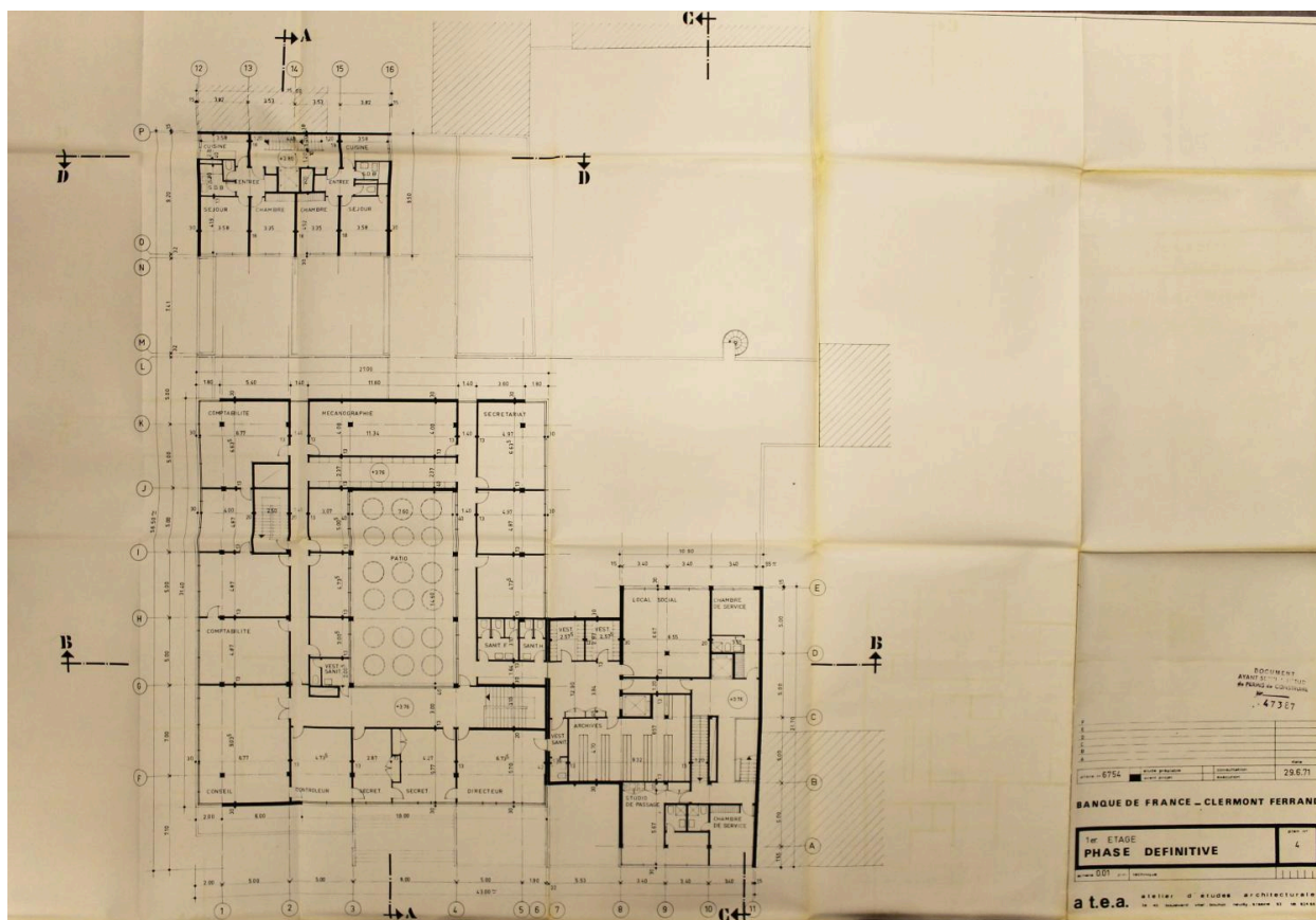
Clermont-Ferrand, succursale de la Banque de France, plan du premier étage, 1971, agence ATEA Lagneau-Weil-Dimitrijevic (Archives municipales de Clermont-Ferrand, 2001 W 296).
