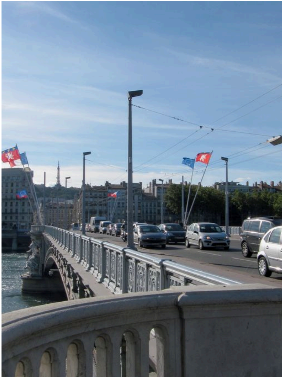
Vue générale, de dessus, chaussée, face aval (depuis la plate-forme de la culée gauche)
