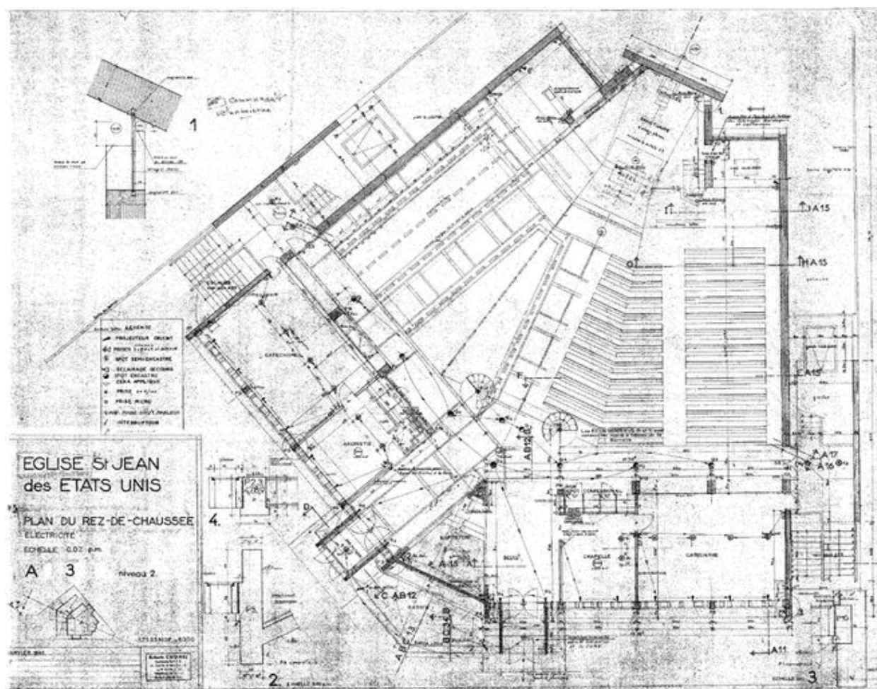
Plan du rez-de-chaussée de l'église, Alain Chomel, 1961
