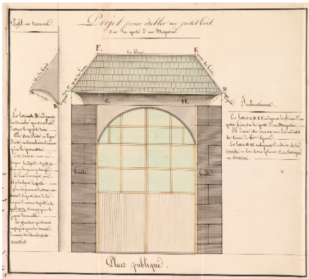
Projet de toit sur la porte d'un magasin
