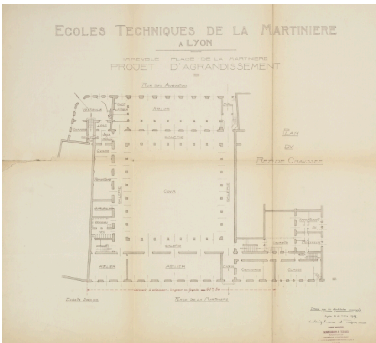
Ecoles techniques de la Martinière. Projet d'agrandissement. Plan du rez-de-chaussée. Document figuré. Plan. Papier. 70 x 60 cm. Archives municipales, Lyon. 344 WP 243 PCA19270346
