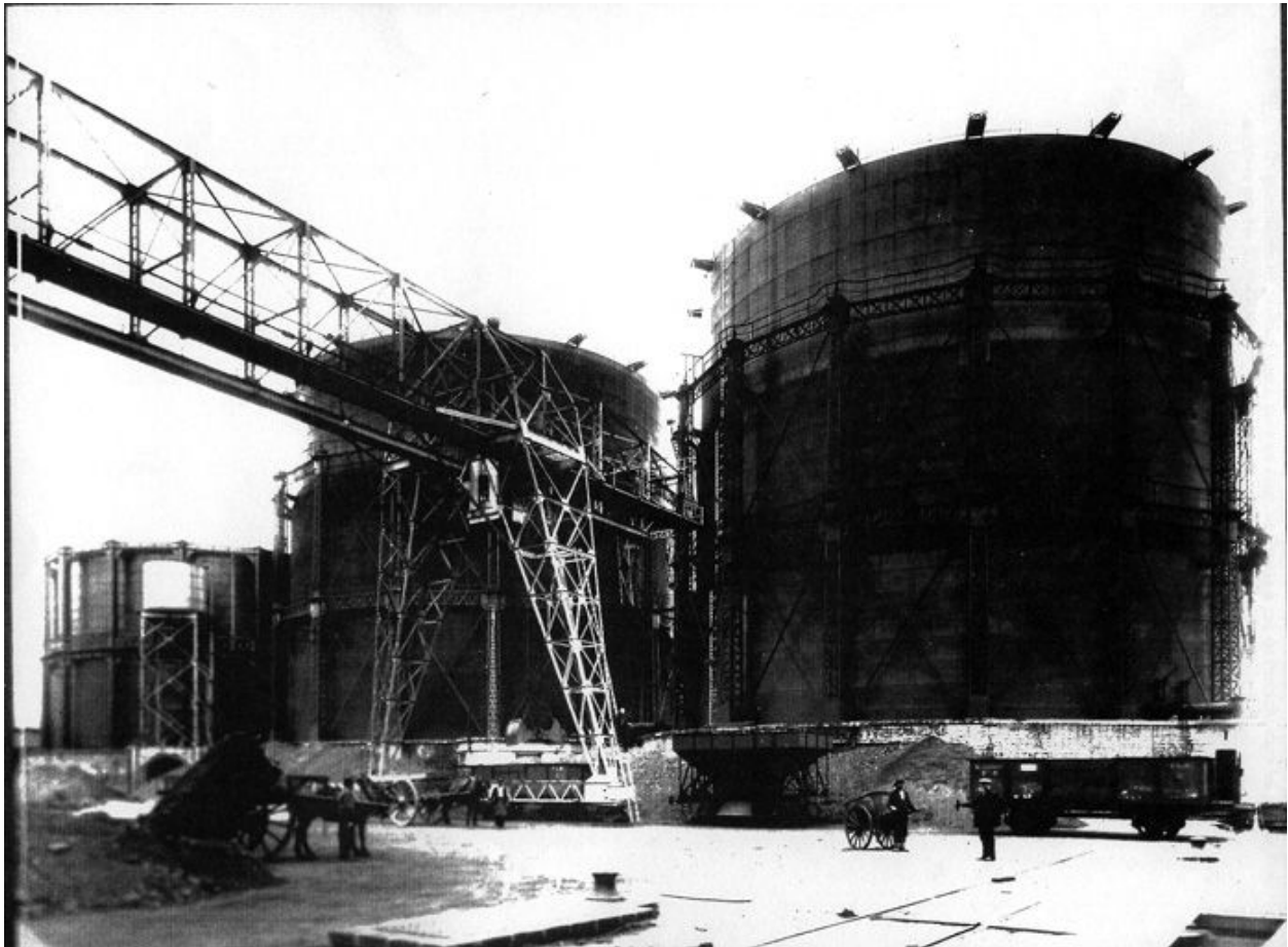
Série de trois gazomètres télescopiques en position haute (1930)
