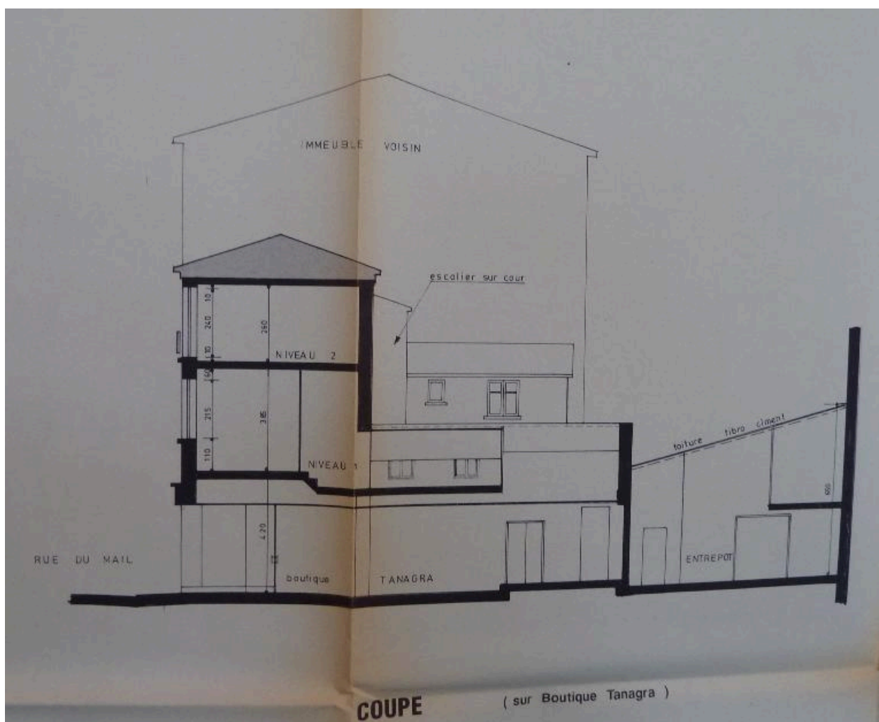
Coupe de l'immeuble avant la restructuration de 1994 (Arch. Mun. Lyon, 1797 W 116 : Permis de construire et de démolir, 1993)
