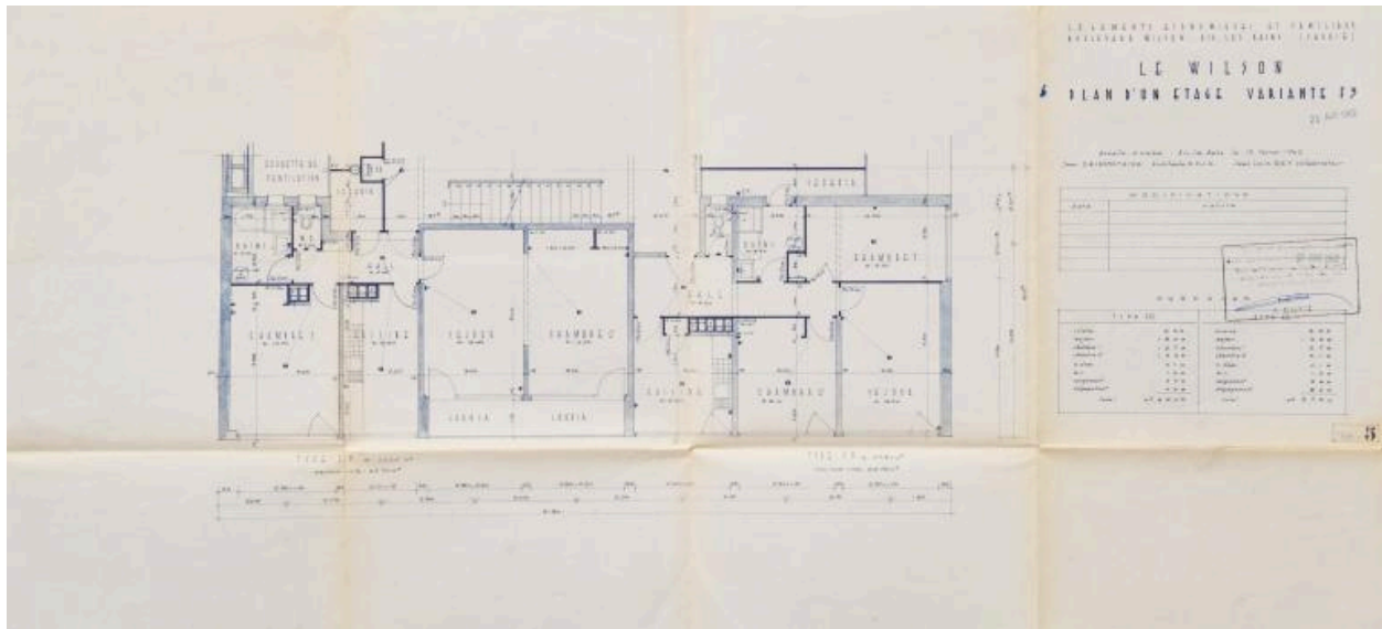
Plan d'un étage, 1962
