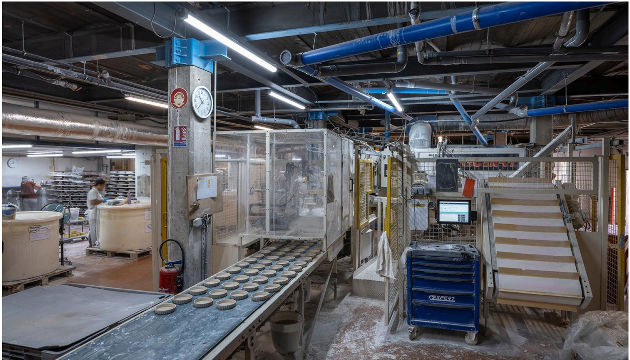
Vue intérieure des ateliers de l'usine de céramique culinaire "Revol porcelaine"
