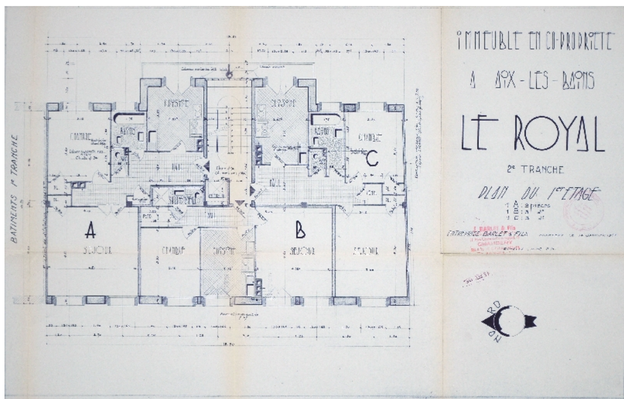
Plan du premier étage
